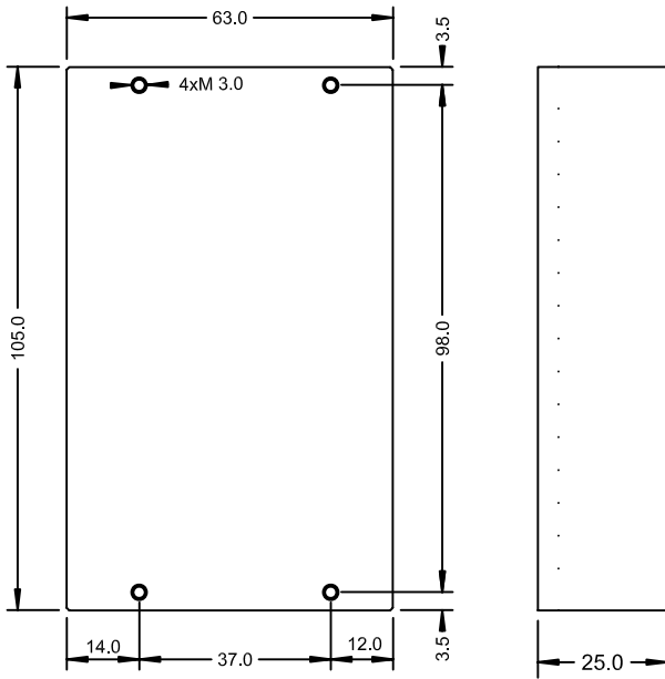
Kühlkörper SK406
